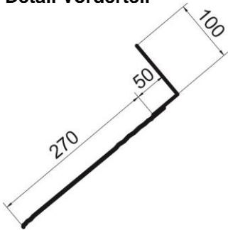
Detail Vorderteil
