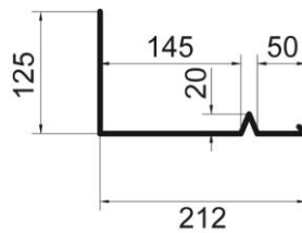
Detail Seitenteil
