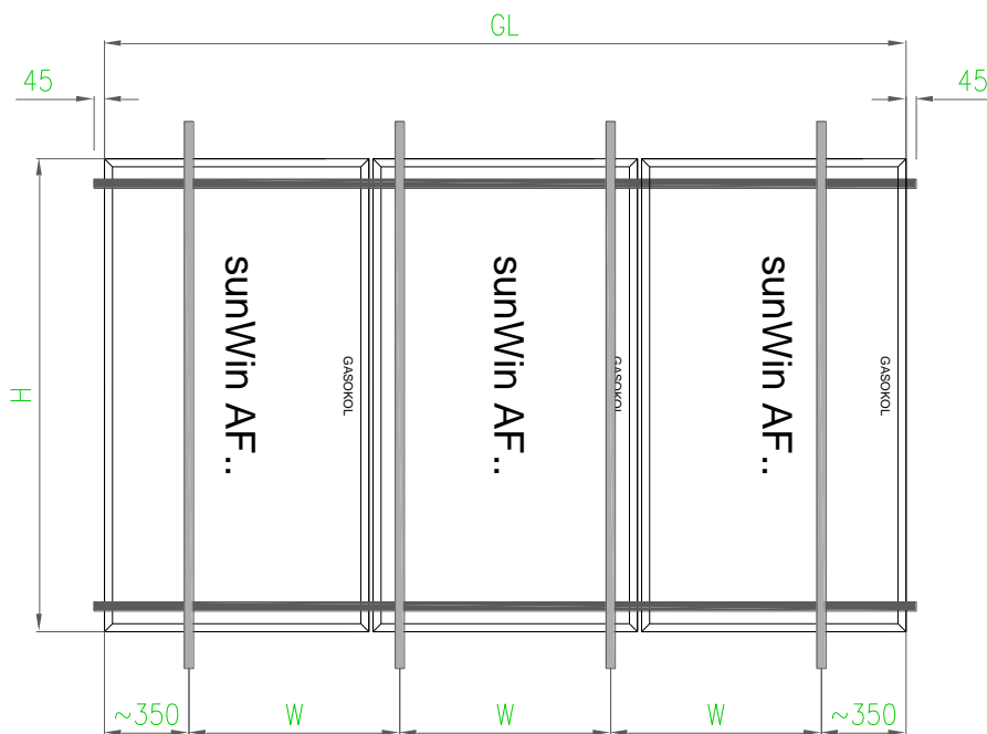
Abbildung Montagesituation, 3 Kollektoren in Reihe
